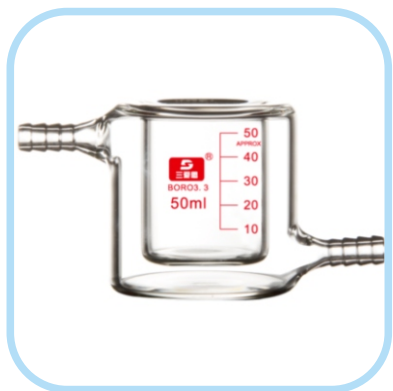
夹套烧杯
