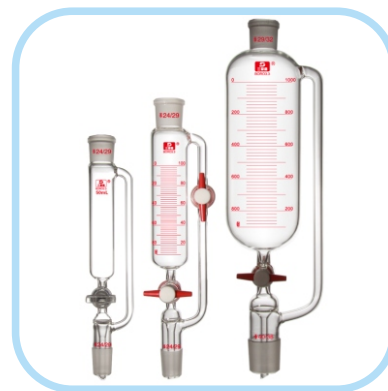
恒压滴液漏斗
